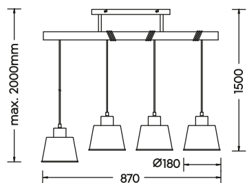
Pendelleuchte · Pendant excl. 4 x E27 max. 40 W 312700432
