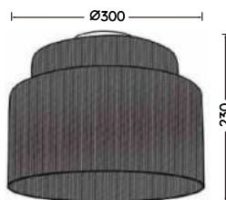
Deckenleuchte · Ceiling lamp excl. 4 x E27 max. 10 W 666800136
