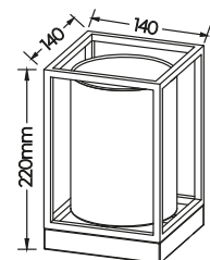
Tischleuchte · Table lamp excl. 1 x E27 max. 25 W 503100144
