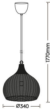
Pendelleuchte · Pendant excl. 1 x E27 max. 10 W 366790136
