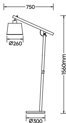
Stehleuchte · Floor lamp excl. 1 x E27 max. 60 W 412700132
