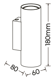
Wandleuchte · Wall lamp excl. 2 x GU10 max. 35 W 212400204
