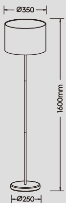
Stehleuchte · Floor lamp excl. 1 x E27 max. 60 W 401100101
