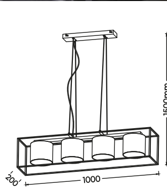
Pendelleuchte · Pendant excl. 4 x E27 max. 25 W 303100417
