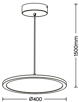
Pendelleuchte · Pendant incl. SMD-LED 29 W / 3.550 Lumen 3.000 Kelvin 340910132
