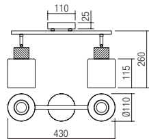
04-528 E27, 2 x max. 42W
