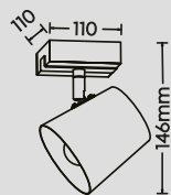
Strahler · Spot excl. 1 x E14 max. 25 W 801900167
