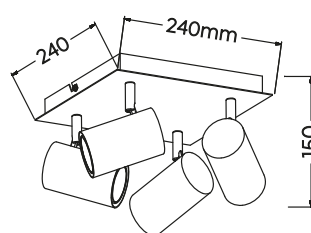
Strahler · Spot excl. 4 x GU10 max. 35 W 802430465
