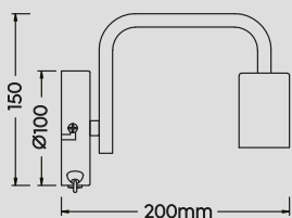
Wandleuchte · Wall lamp excl. 1 x E27 max. 42 W 208070132
