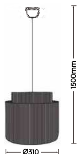
Pendelleuchte · Pendant excl. 1 x E27 max. 10 W 366800136
