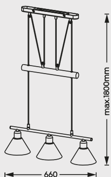
Pendelleuchte · Pendant excl. 3 x E14 max. 40 W 3751031-07
