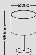
Tischleuchte · Table lamp excl. 1 x E27 max. 40 W 519000144
