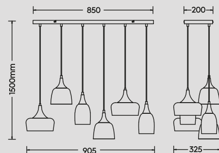
Pendelleuchte · Pendant excl. 6 x E14 max. 25 W 310500632
