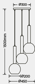
Pendelleuchte · Pendant excl. 3 x E27 max. 28 W 310390332
