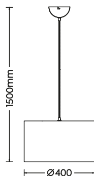
Pendelleuchte · Pendant excl. 1 x E27 max. 60 W 308200179
