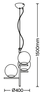
Pendelleuchte · Pendant excl. 3 x E14 max. 28 W 302000308
