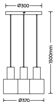
Pendelleuchte · Pendant excl. 3 x E27 max. 40 W 319430317
