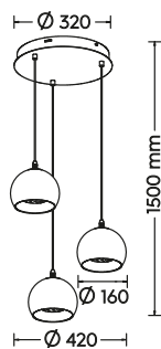
Pendelleuchte · Pendant incl. 3 x SMD-LED 3 x 8 W / 3 x 880 Lumen 2.300 + 3.000 + 4.000 Kelvin 331630306
