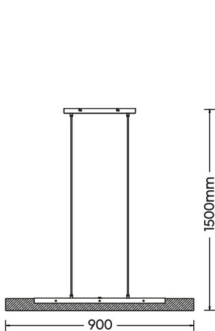
Pendelleuchte · Pendant incl. SMD-LED 25 W / 3.000 Lumen 3.000 Kelvin 341610132
