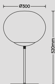
Tischleuchte · Table lamp excl. 1 x E27 max. 15 W 563100108 563100132
