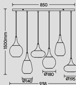
Pendelleuchte · Pendant excl. 6 x E14 max. 40 W 317000613 317000632
