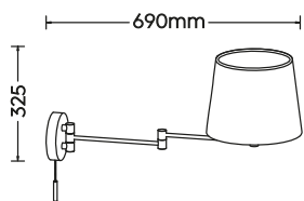
Wandleuchte · Wall lamp excl. 1 x E27 max. 60 W 209100107 209100108
