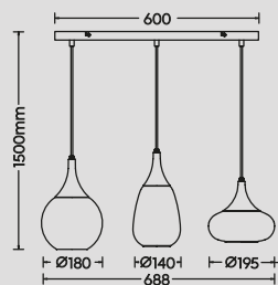
Pendelleuchte · Pendant excl. 3 x E14 max. 40 W 317000313 317000332
