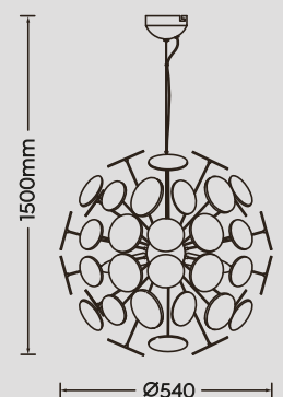
Pendelleuchte · Pendant excl. 6 x E14 max. 40 W 309900657
