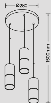
Pendelleuchte · Pendant excl. 3 x E27 max. 40 W 304330332
