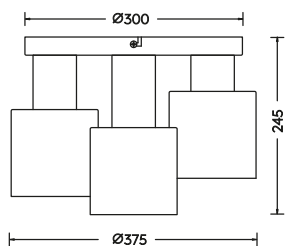
Deckenleuchte · Ceiling lamp excl. 3 x E27 max. 40 W 619430317
