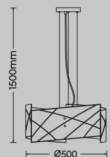
Pendelleuchte · Pendant excl. 3 x E27 max. 40 W 301200300
