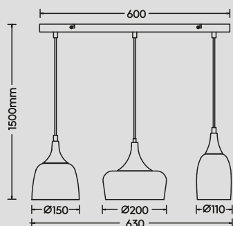
Pendelleuchte · Pendant excl. 3 x E14 max. 25 W 310500332
