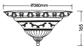
Deckenleuchte · Ceiling lamp excl. 2 x E27 max. 60 W
