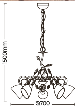
Pendelleuchte · Pendant excl. 5 x E14 max. 40 W 110700528
