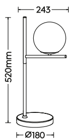
Tischleuchte · Table lamp excl. 1 x E14 max. 28 W 502000108
