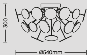
Deckenleuchte · Ceiling lamp
