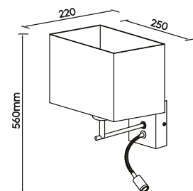
Wandleuchte · Wall lamp
