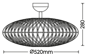
Deckenleuchte · Ceiling lamp excl. 2 x E27 max. 40 W 612300236
