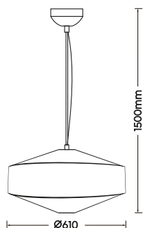
Pendelleuchte · Pendant excl. 1 x E27 max. 10 W 364790144
