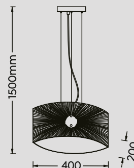
Pendelleuchte · Pendant excl. 2 x E27 max. 40 W 312200200
