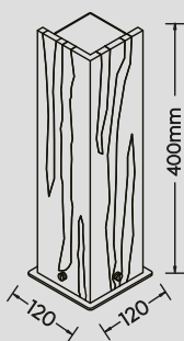
Tischleuchte · Table lamp excl. 1 x E27 max. 10 W 563300130
