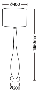
Stehleuchte · Floor lamp excl. 1 x E27 max. 10 W 467200130
