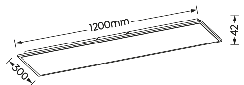
Deckenleuchte · Ceiling lamp incl. SMD-LED 31 W / 3.600 Lumen 3.000 Kelvin 674011207
