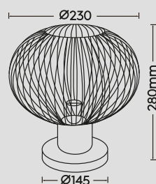
Tischleuchte · Table lamp excl. 1 x E27 max. 10 W 565700132 565700166
