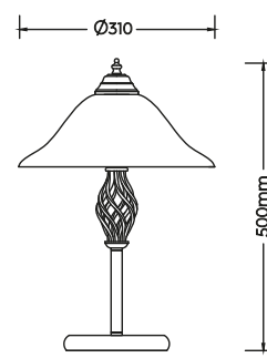
Tischleuchte · Table lamp excl. 2 x E14 max. 40 W 501000224
