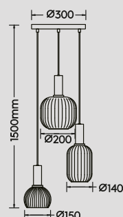
Pendelleuchte · Pendant excl. 3 x E27 max. 10 W 319830308 319830332
