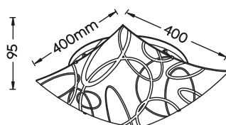
Deckenleuchte · Ceiling lamp excl. 2 x E27 max. 40 W 604400201
