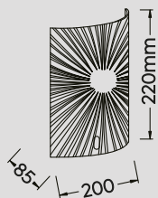
Wandleuchte · Wall lamp excl. 1 x E27 max. 40 W 212200100
