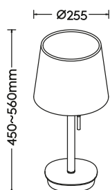
Tischleuchte · Table lamp excl. 1 x E27 max. 60 W 509100107 509100108
