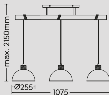
Pendelleuchte · Pendant excl. 3 x E27 max. 42 W 303400367
