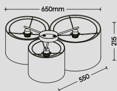
Deckenleuchte · Ceiling lamp excl. 3 x E27 max. 40 W 611490332
