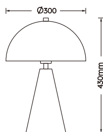
Tischleuchte · Table lamp excl. 1 x E27 max. 40 W 565000132 565000176
