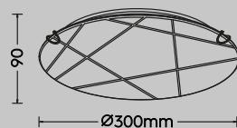
Deckenleuchte · Ceiling lamp excl. 1 x E27 max. 40 W 601200100
