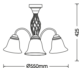
Deckenleuchte · Ceiling lamp excl. 3 x E14 max. 40 W 601000324
