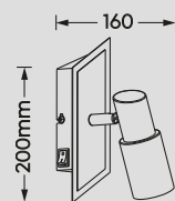
Strahler · Spot incl. SMD-LED 1 x 4,3 W / 1 x 430 Lumen 3.000 Kelvin 821470105
