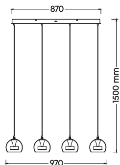
Pendelleuchte · Pendant incl. 4 x SMD-LED 4 x 8 W / 4 x 880 Lumen 2.300 + 3.000 + 4.000 Kelvin 331610406
