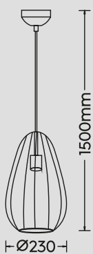
Pendelleuchte · Pendant excl. 1 x E27 max. 10 W 365300104
