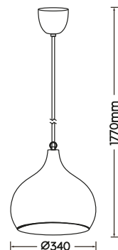
Pendelleuchte · Pendant excl. 1 x E27 max. 10 W 366790136
