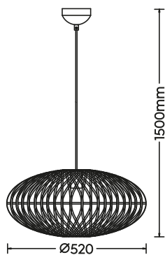
Pendelleuchte · Pendant excl. 1 x E27 max. 40 W 312300136
