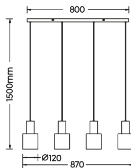
Pendelleuchte · Pendant excl. 4 x E27 max. 40 W 319400417
