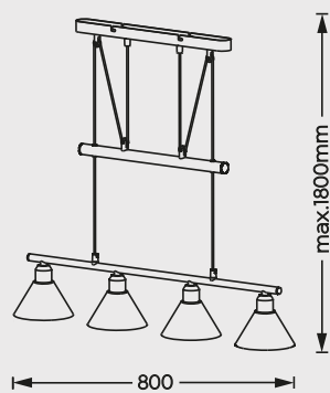
Pendelleuchte · Pendant excl. 4 x E14 max. 40 W 3751041-07
