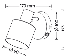
Strahler · Spot excl. 1 x E14 max. 10 W 868870180
