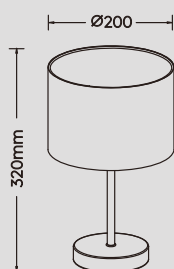
Tischleuchte · Table lamp excl. 1 x E14 max. 40 W 501100101
