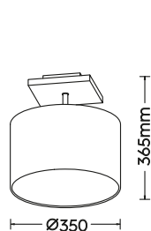
Deckenleuchte · Ceiling lamp excl. 1 x E27 max. 60 W 602100130
