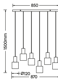
Pendelleuchte · Pendant excl. 6 x E27 max. 40 W 319400617
