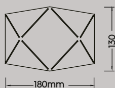
Wandleuchte · Wall lamp incl. SMD-LED 6,5 W / 700 Lumen 3.000 Kelvin 223510131
