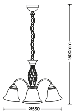
Pendelleuchte · Pendant excl. 3 x E14 max. 40 W 101000324
