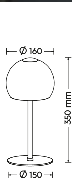
Tischleuchte · Table lamp incl. SMD-LED 8 W / 880 Lumen 2.300 + 3.000 + 4.000 Kelvin 531610106
