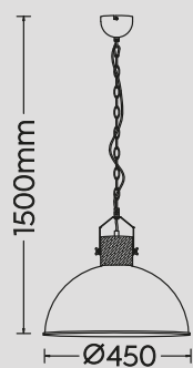
Pendelleuchte · Pendant excl. 1 x E27 max. 60 W 303400167
