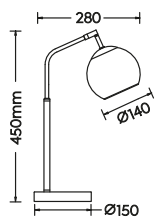
Tischleuchte · Table lamp
