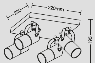
Strahler · Spot excl. 4 x E14 max. 40 W 804300432
