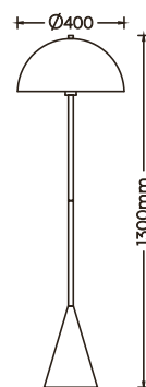
Stehleuchte · Floor lamp excl. 1 x E27 max. 40 W 465000132 465000176
