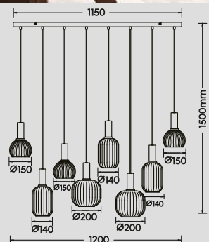
Pendelleuchte · Pendant excl. 8 x E27 max. 10 W 319800808 319800832
