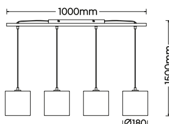
Pendelleuchte · Pendant excl. 4 x E27 max. 60 W 302100430
