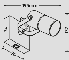
Strahler · Spot excl. 1 x E14 max. 15 W 804370132
