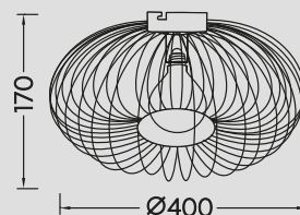
Deckenleuchte · Ceiling lamp excl. 1 x E27 max. 60 W 606900132 606900162
