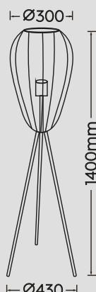
Stehleuchte · Floor lamp excl. 1 x E27 max. 10 W 465300104
