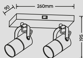
Strahler · Spot excl. 2 x E14 max. 15 W 804370232
