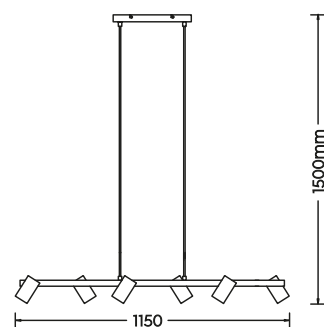
Pendelleuchte · Pendant excl. 6 x GU10 max. 35 W 312490632
