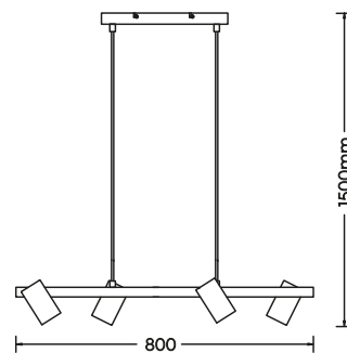
Pendelleuchte · Pendant excl. 4 x GU10 max. 35 W 302400432
