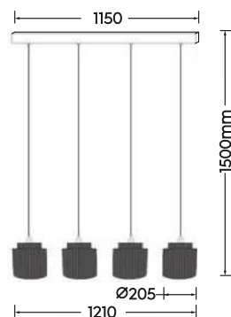
Pendelleuchte · Pendant excl. 4 x E27 max. 10 W 366800436
