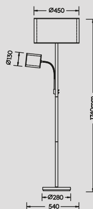
Stehleuchte · Floor lamp excl. 1 x E27, max. 60 W excl. 1 x E14, max. 40 W 411400232
