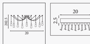
Squiggle- 9Lt Pendant Black Metal & Cable
