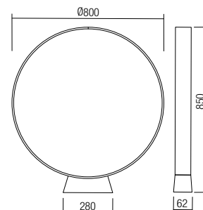
BOLLARD • STÂLPÎSOR • Ø800
