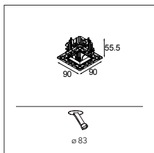
QBINI TRIMLESS FRAME 1X
