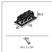
QBINI TRIMLESS FRAME 3X
